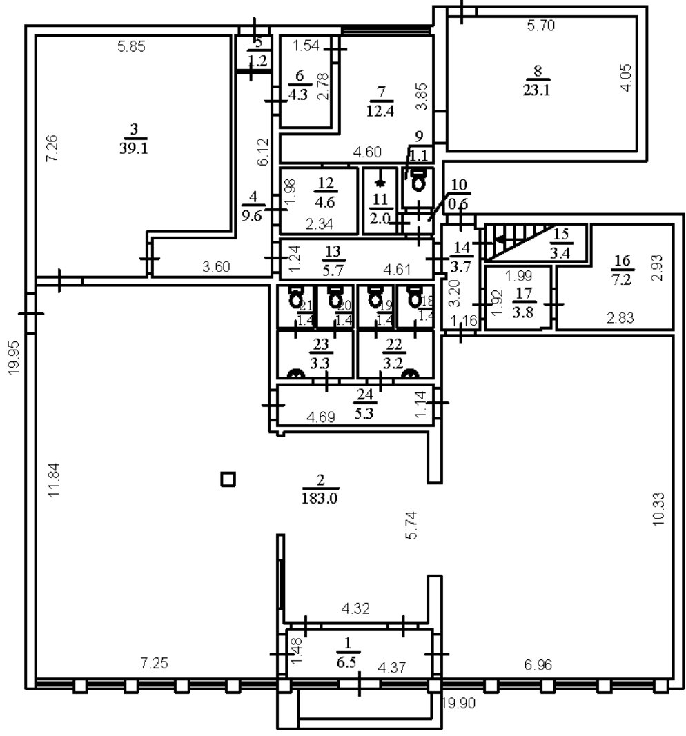
ПІДВАЛ ПІД ЛІТ. "А"
